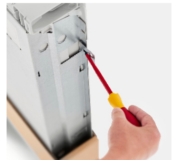
08 Befestigungslasche zur Befestigung im Mauerwerk
