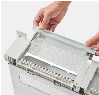
09 Herausnehmbarer Leitungseinführungsschieber zum schnellen Einführen der Leitungen; pro Feldbreite je ein Schieber oben und unten
