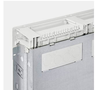
12 Rückwärtige und seitliche Leitungseinführungsmöglichkeiten
