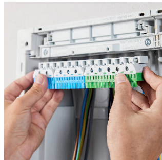
11 Die Klemmschienen mit den N/PE Quick-Steckklemmen werden einfach von vorne eingeklickt; zusätzlich können die Leitungen an der Kabelabfang-/Zugentlastungsbefestigung fixiert werden
