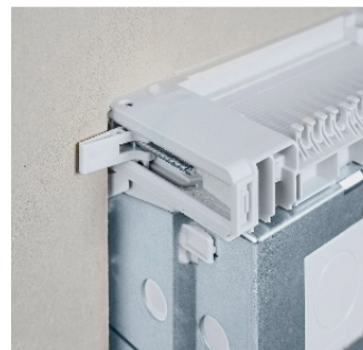
07 Stabile Befestigung durch Hohlwandkrallen
