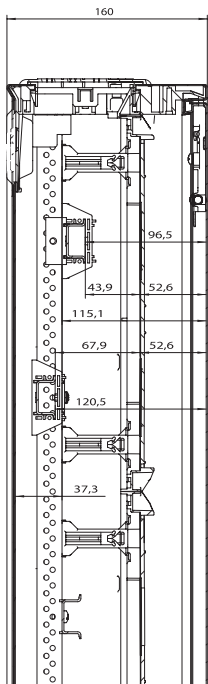
Klemmenfeld
