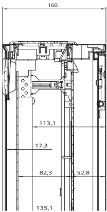
Montageplattenfeld
